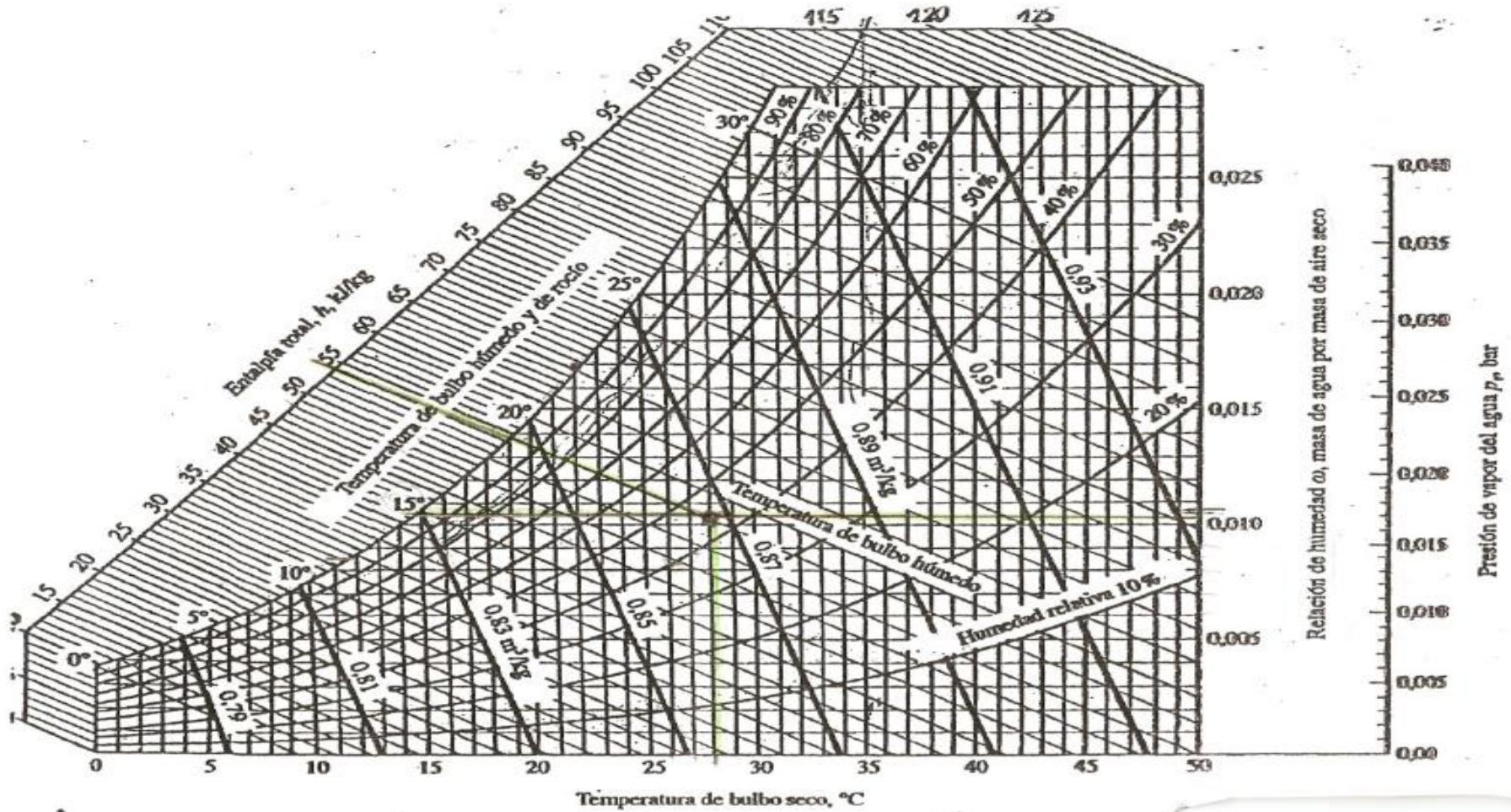
Figura A.25. Diagrama psicrométrico, unidades métricas, presión barométrica 1,01 bar.
