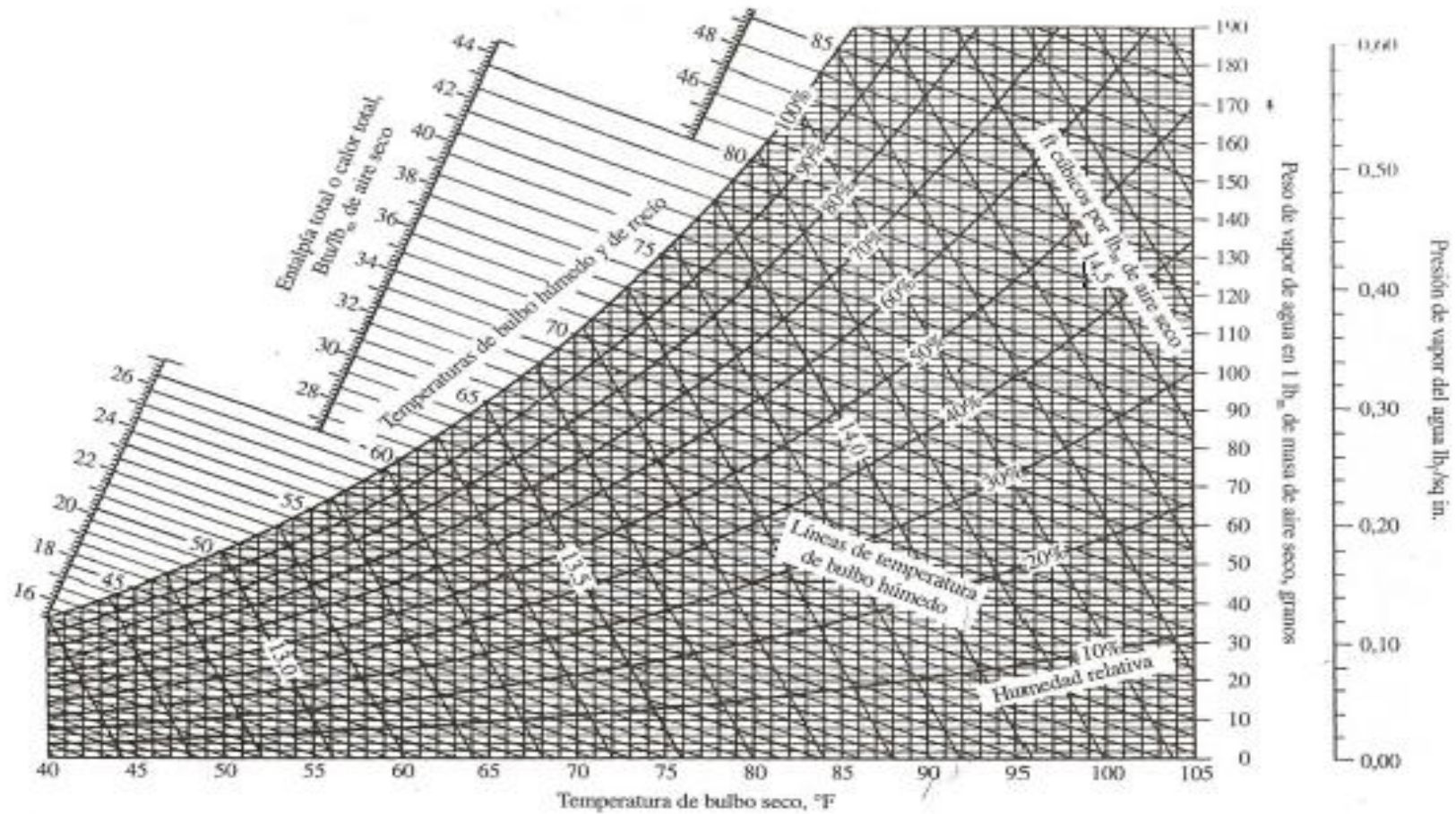
Figura A.25I. Diagrama psicrométrico, unidades USCS, presión barométrica 14,696 psia (Copyright, 1942, por General Electric Company).
